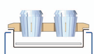
Kompletter Zusammenbau, in den Werkzeugrahmen eingesetzt
